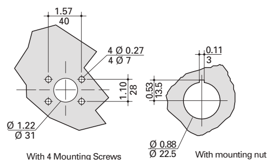
Door drilling layouts
