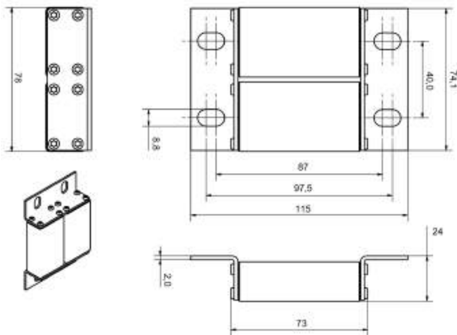
Size 230
