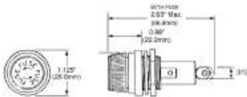
HPD
