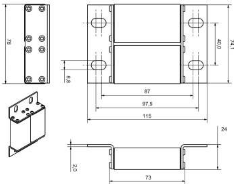
Size 230
