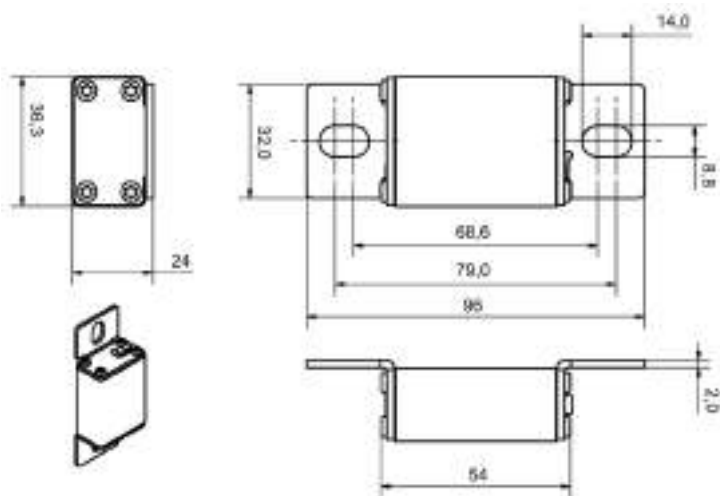
Size 000
