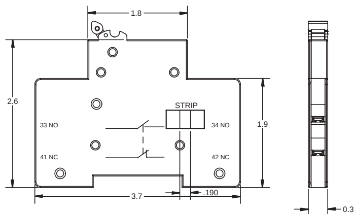
CCP2-AUX
