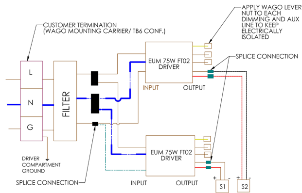
11-UNV1-SG1-S892 / 13-UNV1-SG1-S892-M2
