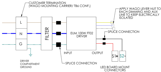
11-UNV1-SG1 / 13-UNV1-SG1-M2
