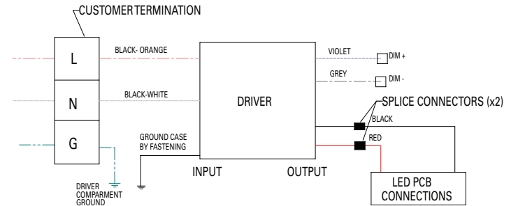
3 - 5 - 7 - 9 - 11 - UNV34 / 13-UNV34-M2
