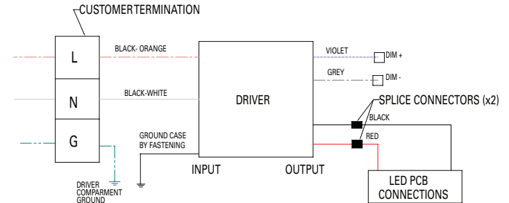
3 - 5 - 7 - 9 - 11 - UNV34 / 13-UNV34-M2
