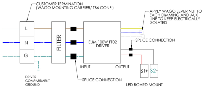
11-UNV1-SG1 / 13-UNV1-SG1-M2
