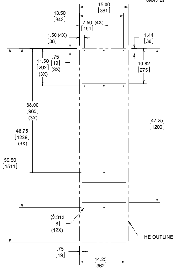
Cutout Dimensions
