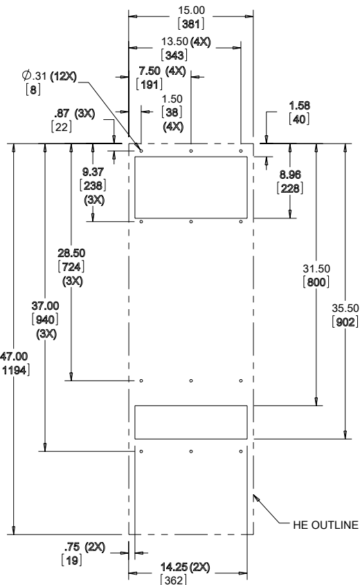
Cutout Dimensions
