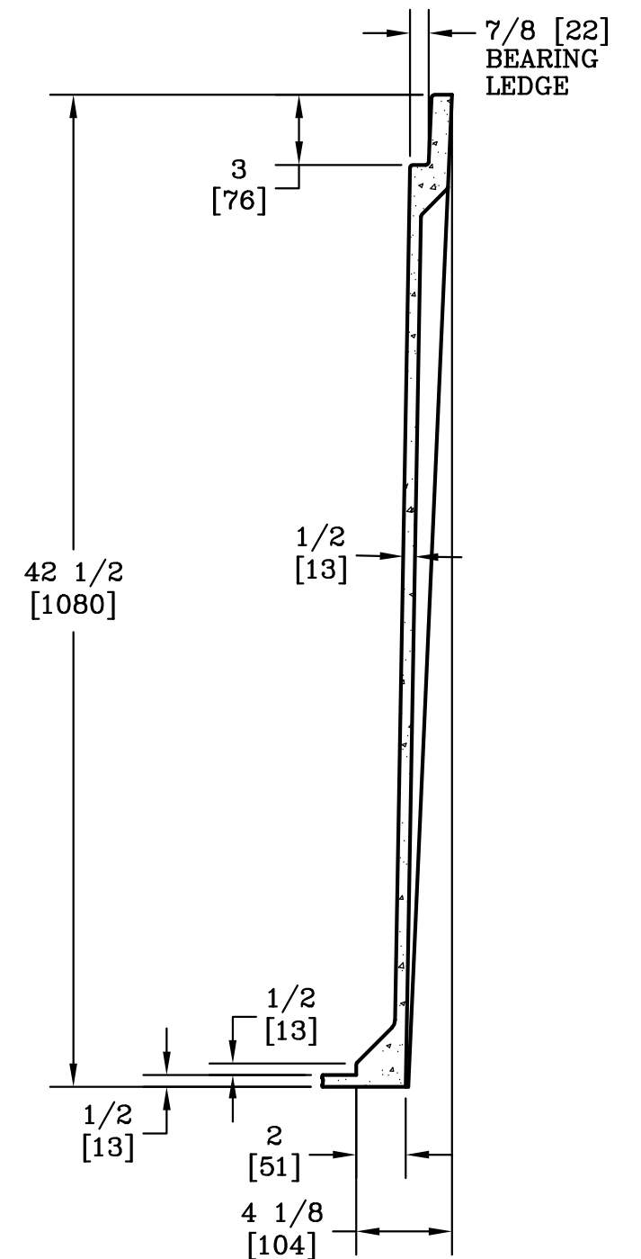
SECTION A-A SCALE: 1 1/2"=1'
