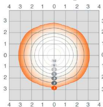
LNHIBA2A-300UNVD840-24W_20FT
