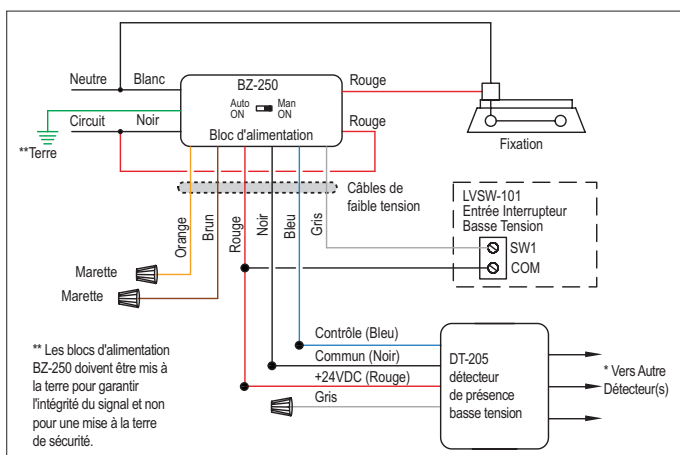
Câblage de la marche manuelle avec un interrupteur instantané basse tension
