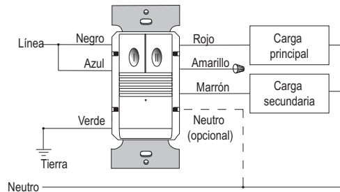
PW-302 y PW-302-347 Cableado de dos niveles
