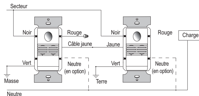
Câblage standard (PW-301 ou PW-301-347 - jusqu'à 4 détecteurs)
