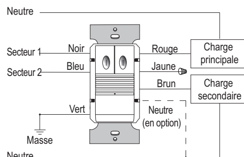
Câblage à double circuit des PW-302 et PW-302-347
