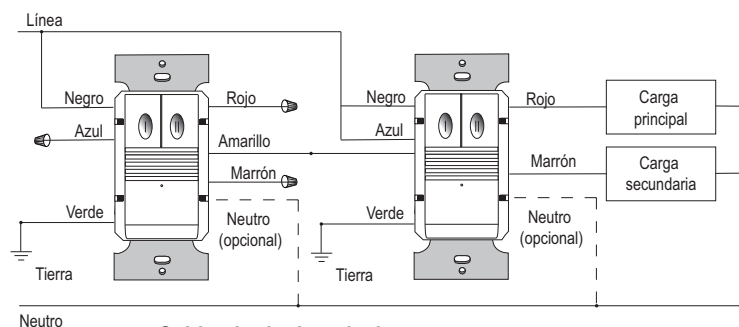
Cableado de dos niveles (PW-302 o PW-302-347 – hasta 4 sensores)
