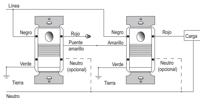
Cableado típico (PW-301 o PW-301-347 – hasta 4 sensores)
