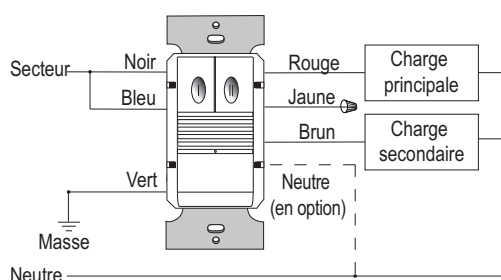
Câblage à deux niveaux des PW-302 et PW-302-347
