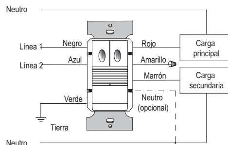
Cableado en dos fases
