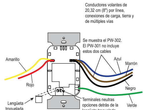
PW-302 y PW-302-347 Cableado de dos circuitos
