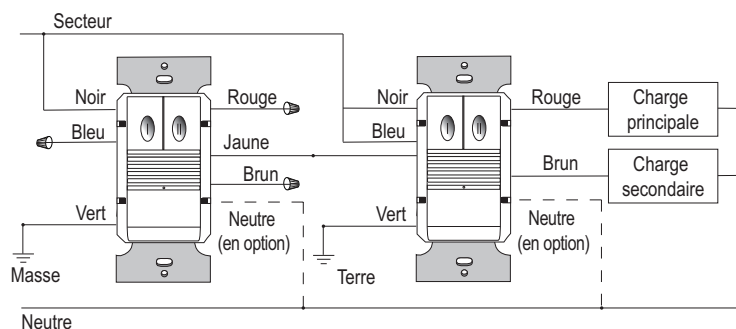
Câblage à deux niveaux (PW-302 ou PW-302-347 - jusqu'à 4 détecteurs)
