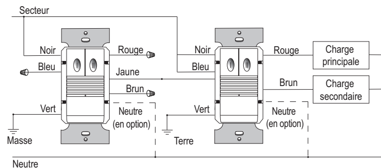
Câblage biphase
