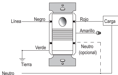
Cableado de PW-301 y PW-301-347
