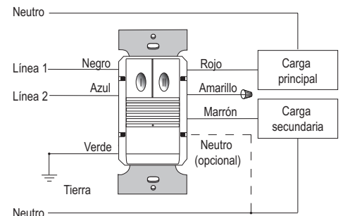
PW-302 y PW-302-347 Cableado de dos circuitos
