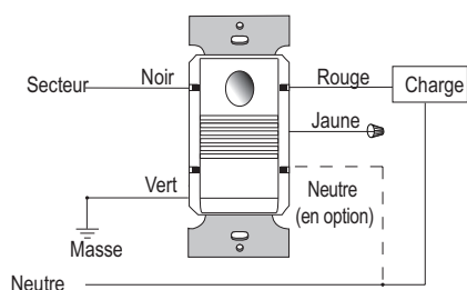
Câblage des PW-301 et PW-301-347
